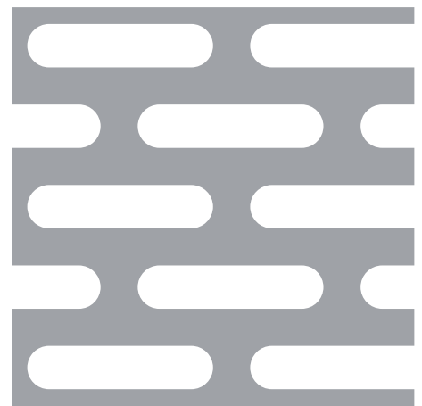
TOT 7x30mm - 26x36 / AA 42,6%
